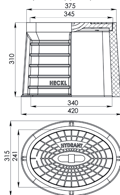
Hydrantový poklop
