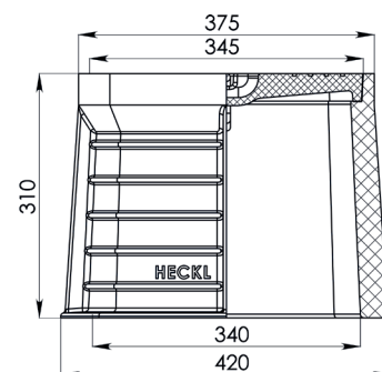
Hydrantový poklop
