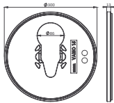
Deska Vario 15 plastová
